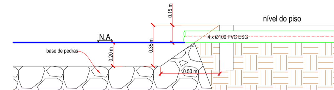
DETALHE 0 Corte - Entrada de água Esc.: 1:20
