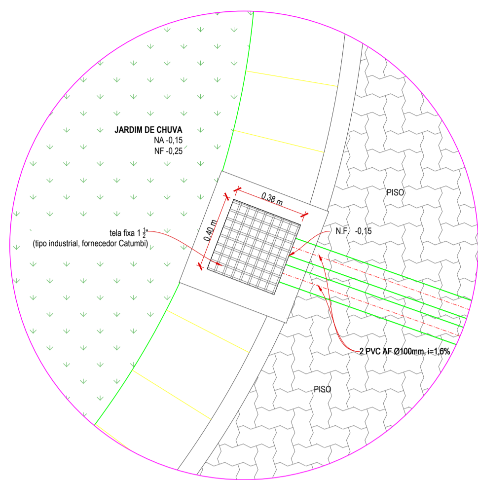
DETALHE 1 Planta - Caixa de saída de água (ladrão) Esc.: 1:20
