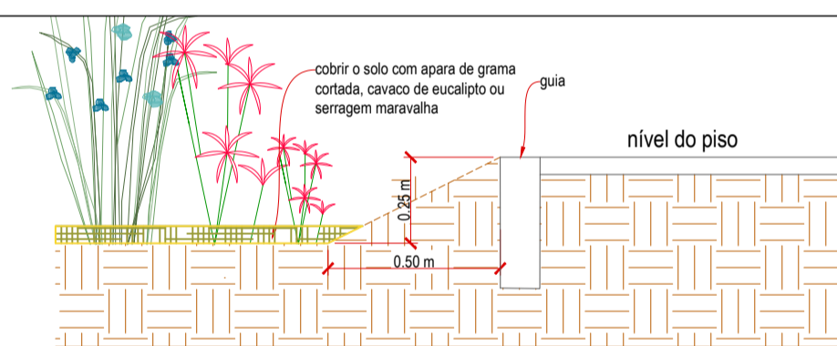
DETALHE 1 Corte - Terreno Esc.: 1:20
