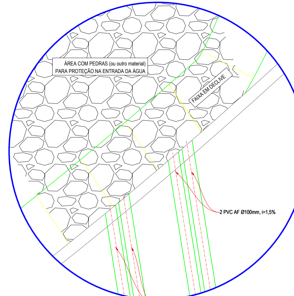
DETALHE 0 Planta - Entrada de água da rua Esc.: 1:20
