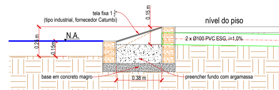
DETALHE 1 Corte - Caixa de saída de água (ladrão) Esc.: 1:20
