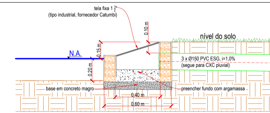
DETALHE 3 Corte - Caixa de saída de água (ladrão) Esc.: 1:20
