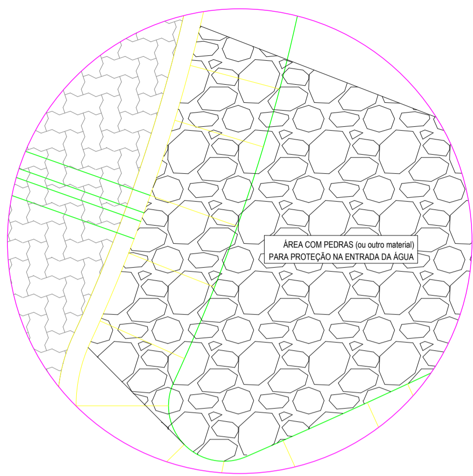
DETALHE 2 Planta - Caixa de saída de água (ladrão) Esc.: 1:20
