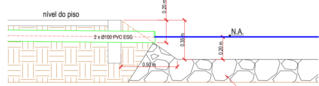
DETALHE 2 Corte - Entrada de água Esc.: 1:20
