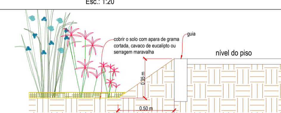
DETALHE 3 Corte - Terreno Esc.: 1:20
