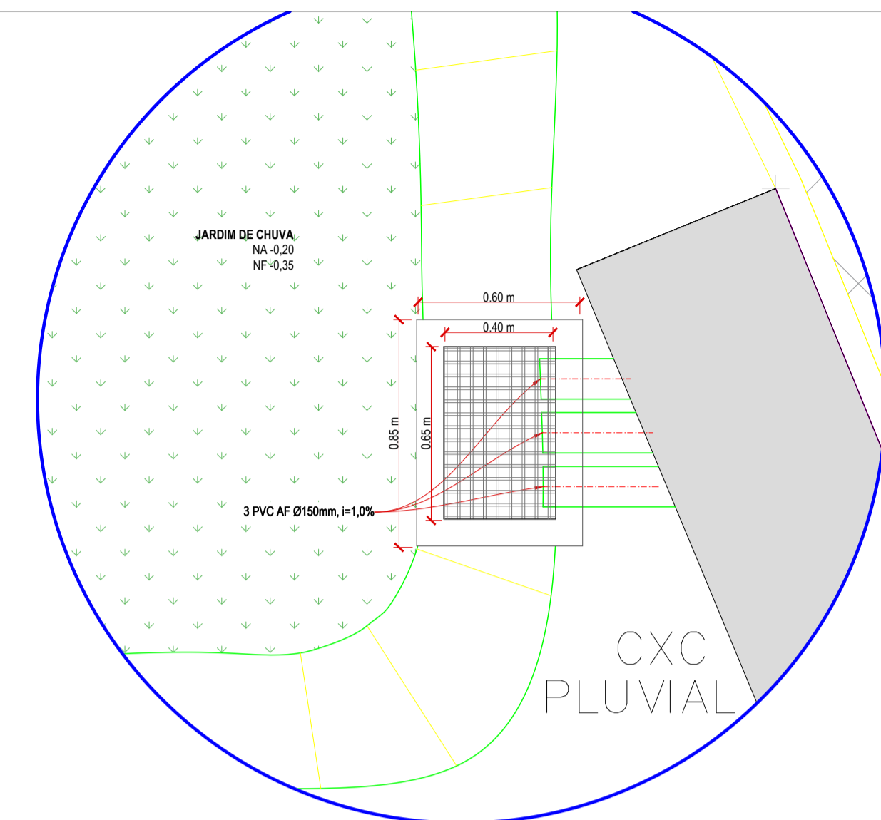
DETALHE 3 Planta - Caixa de saída de água (ladrão final) Esc.: 1:20
